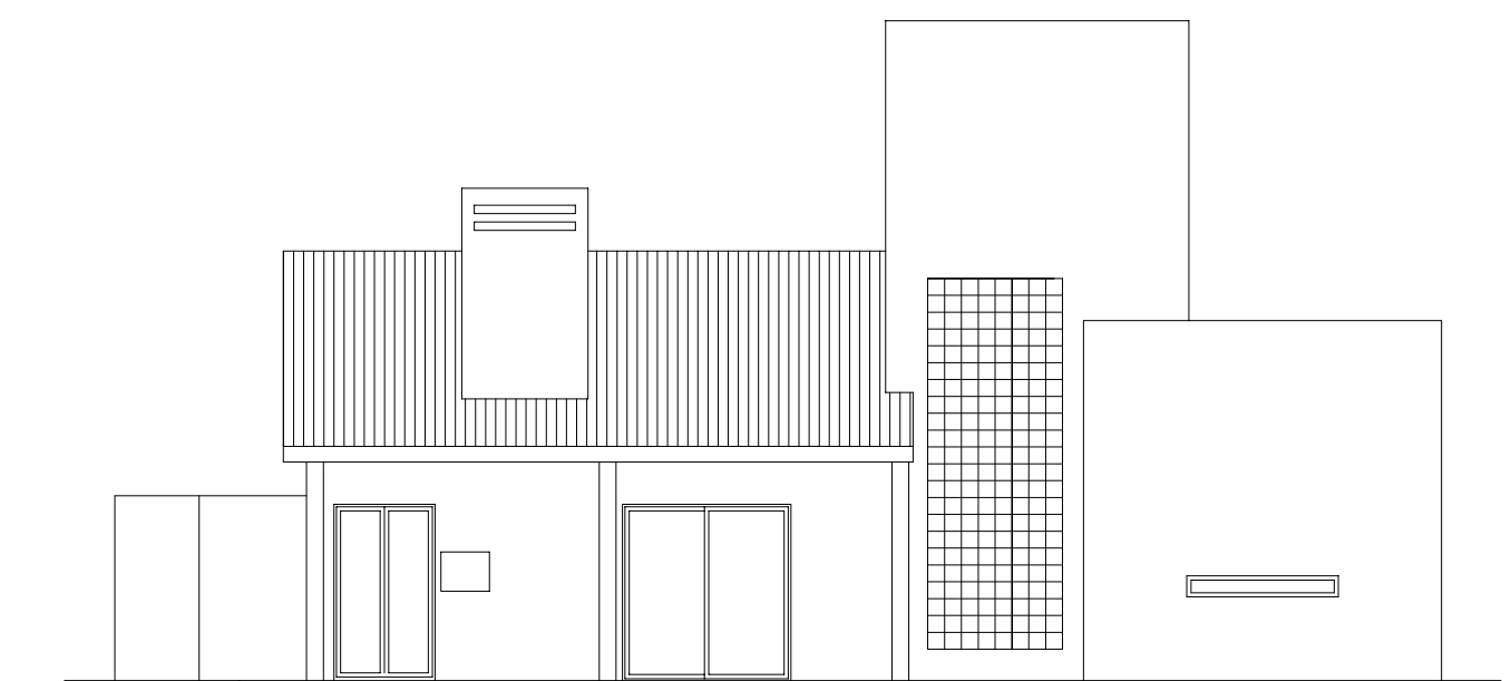
ALZADO A LA MARISMA
