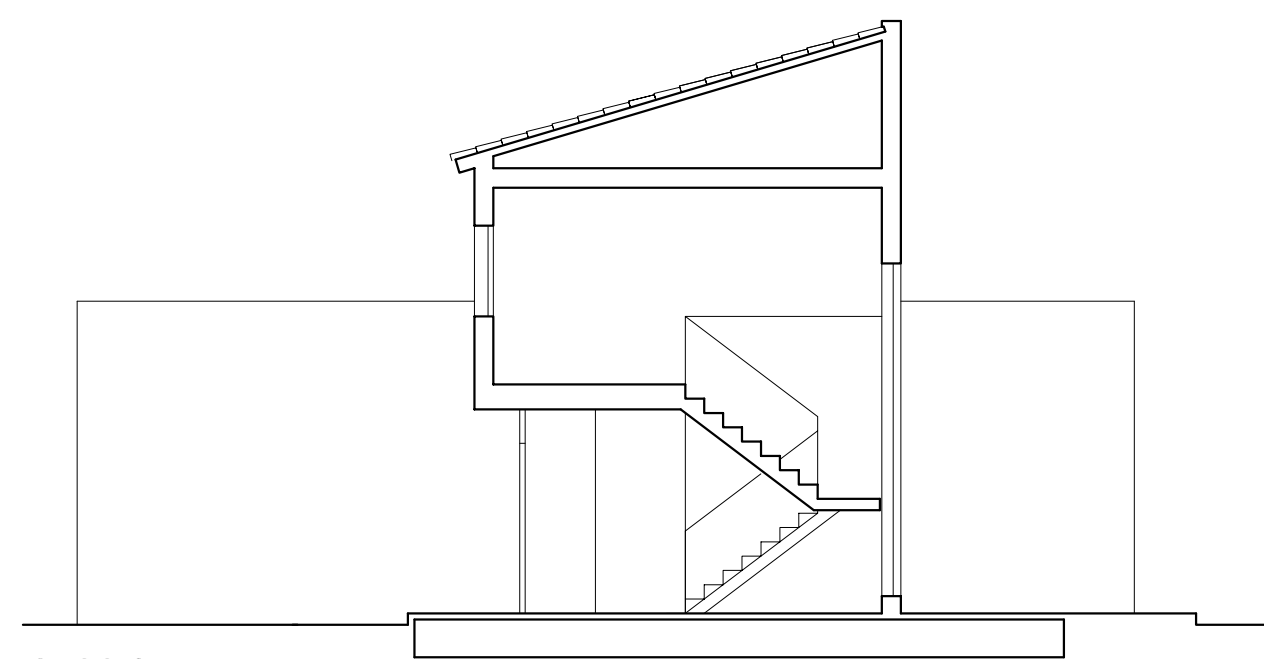
SECCION A-A
