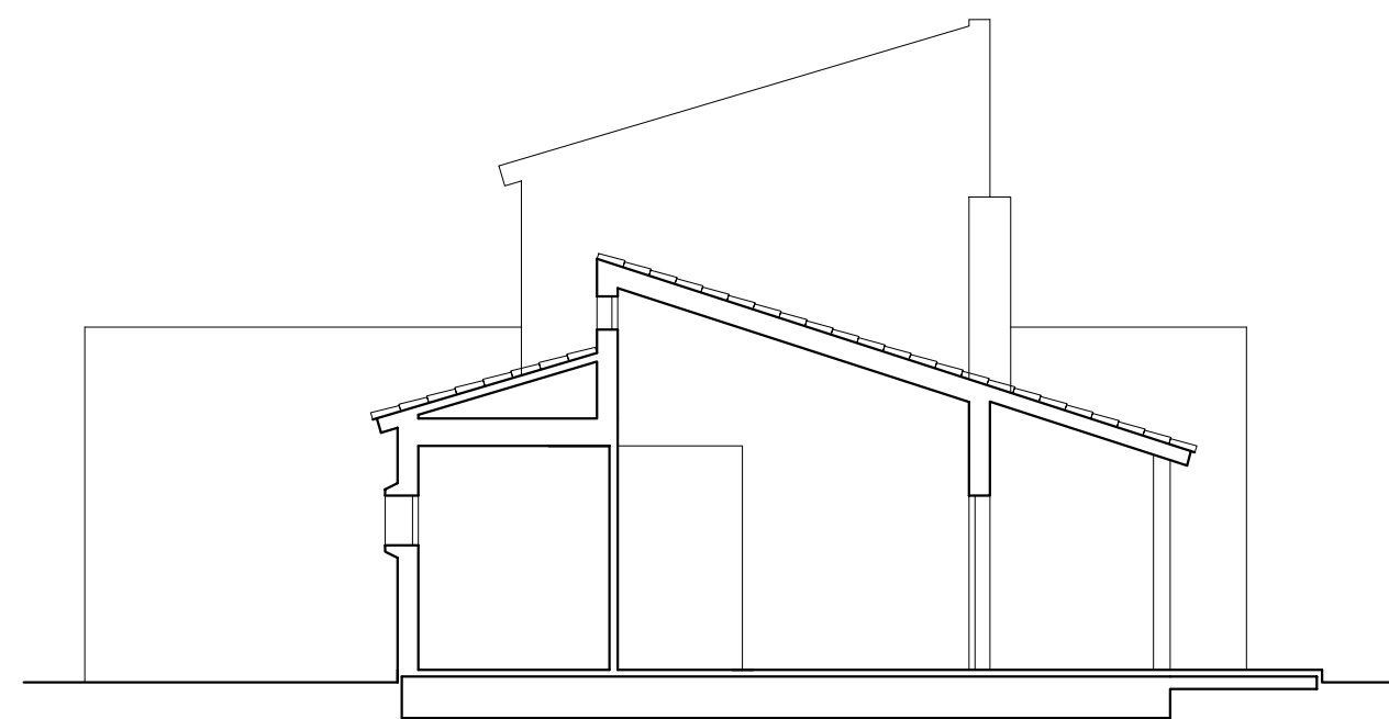
SECCION B-B
